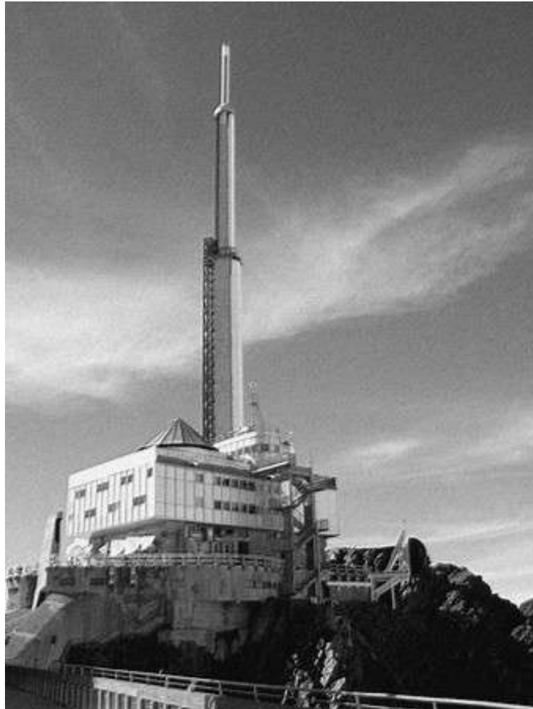
Proche de Tarbes, l'Observatoire du Pic du Midi, qui avec son télescope géant, a permis au début des années 60, de préparer les missions Apollo, vers la Lune
